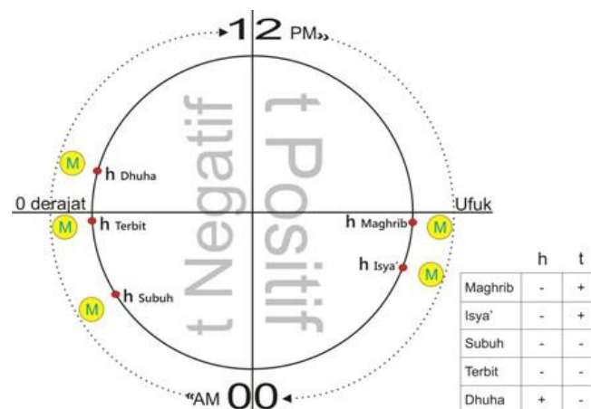
Gambar hubungan tinggi matahari dan sudut waktu
